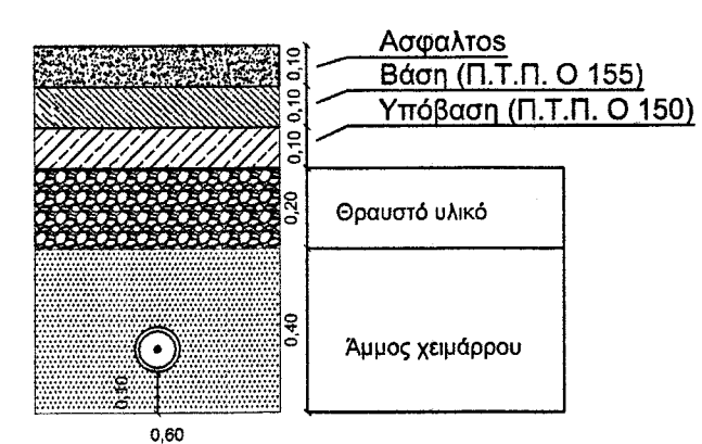
ΤΥΠΙΚΗ ΔΙΑΤΟΜΗ 1 ΟΔΕΥΣΗ ΕΝΟΣ ΑΓΩΓΟΥ ΕΝΤΟΣ/ΕΚΤΟΣ ΟΙΚΙΣΜΟΥ ΕΠΙ ΑΣΦΑΛΤΟΣΤΡΩΜΕΝΗΣ ΟΔΟΥ
