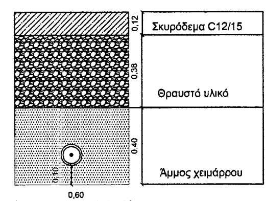
ΤΥΠΙΚΗ ΔΙΑΤΟΜΗ 2 ΟΔΕΥΣΗΣ ΑΓΩΓΟΥ ΕΝΤΟΣ/ΕΚΤΟΣ ΟΙΚΙΣΜΟΥ ΕΠΙ ΤΣΙΜΕΝΟΣΤΡΩΜΕΝΗΣ ΟΔΟΥ
