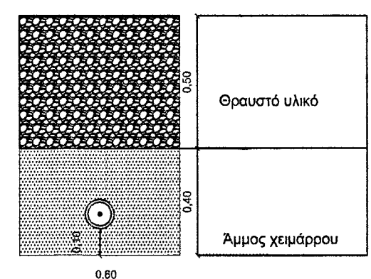
ΤΥΠΙΚΗ ΔΙΑΤΟΜΗ 3 ΟΔΕΥΣΗΣ ΑΓΩΓΟΥ ΕΝΤΟΣ/ΕΚΤΟΣ ΟΙΚΙΣΜΟΥ ΕΠΙ ΧΑΛΙΚΟΣΤΡΩΜΕΝΗΣ ΟΔΟΥ
