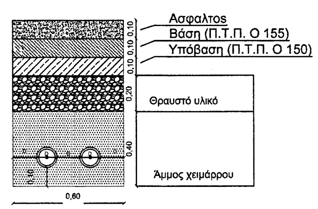
ΤΥΠΙΚΗ ΔΙΑΤΟΜΗ 1 ΟΔΕΥΣΗ ΔΥΟ ΑΓΩΓΩΝ ΕΝΤΟΣ/ΕΚΤΟΣ ΟΙΚΙΣΜΟΥ ΕΠΙ ΑΣΦΑΛΤΟΣΤΡΩΜΕΝΗΣ ΟΔΟΥ
