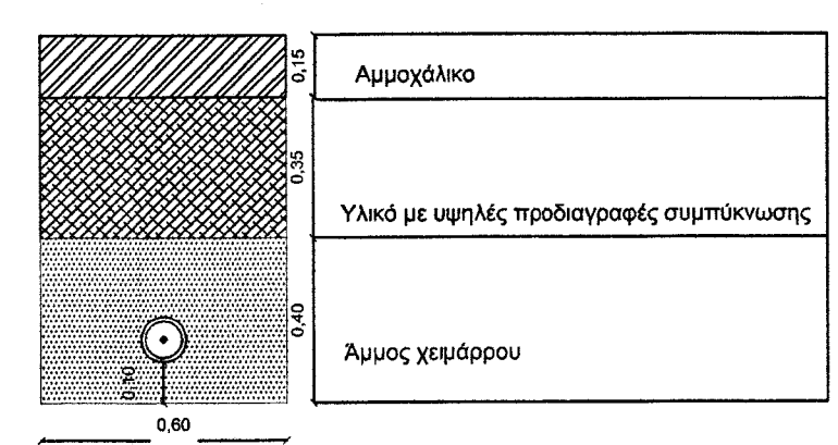
ΤΥΠΙΚΗ ΔΙΑΤΟΜΗ 6 ΟΔΕΥΣΗ ΕΝΟΣ ΑΓΩΓΟΥ ΕΚΤΟΣ/ΕΚΤΟΣ ΟΙΚΙΣΜΟΥ ΕΠΙ ΧΑΛΙΚΟΣΤΡΩΜΕΝΗΣ ΑΓΡΟΤΙΚΗΣ ΟΔΟΥ
