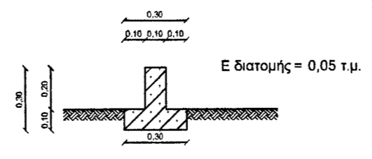
ΛΕΠΤΟΜΕΡΕΙΑ - Τομή α-α Κλίμακα 1:25
