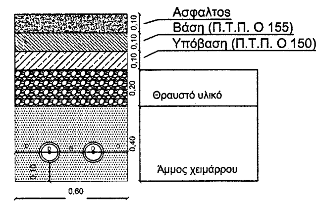
ΤΥΠΙΚΗ ΔΙΑΤΟΜΗ 1 ΟΔΕΥΣΗ ΔΥΟ ΑΓΩΓΩΝ ΕΝΤΟΣ ΟΙΚΙΣΜΟΥ ΕΠΙ ΑΣΦΑΛΤΟΣΤΡΩΜΕΝΗΣ ΟΔΟΥ
