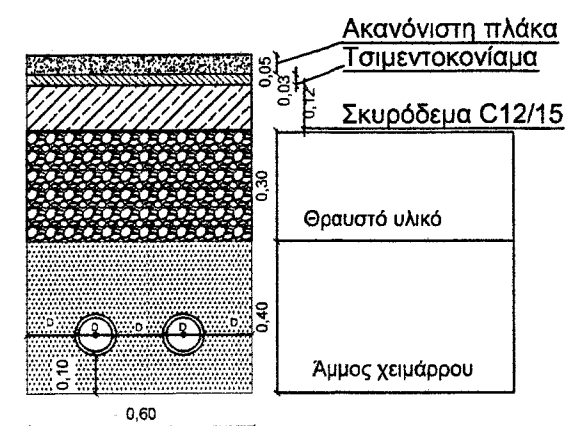
ΤΥΠΙΚΗ ΔΙΑΤΟΜΗ 5 ΟΔΕΥΣΗ ΔΥΟ ΑΓΩΓΩΝ ΕΝΤΟΣ ΟΙΚΙΣΜΟΥ ΕΠΙ ΠΛΑΚΟΣΤΡΩΜΕΝΗΣ ΟΔΟΥ
