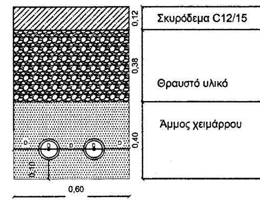
ΤΥΠΙΚΗ ΔΙΑΤΟΜΗ 2 ΟΔΕΥΣΗ ΔΥΟ ΑΓΩΓΩΝ ΕΝΤΟΣ ΟΙΚΙΣΜΟΥ ΕΠΙ ΤΣΙΜΕΝΟΣΤΡΩΜΕΝΗΣ ΟΔΟΥ
