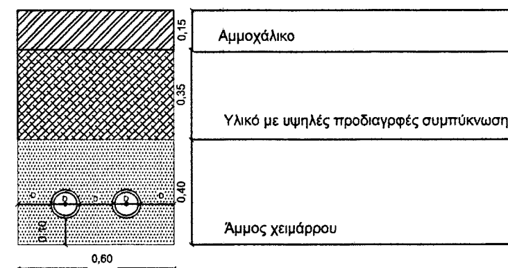
ΤΥΠΙΚΗ ΔΙΑΤΟΜΗ 6 ΟΔΕΥΣΗ ΔΥΟ ΑΓΩΓΩΝ ΕΚΤΟΣ ΟΙΚΙΣΜΟΥ ΕΠΙ ΧΑΛΙΚΟΣΤΡΩΜΕΝΗΣ ΑΓΡΟΤΙΚΗΣ ΟΔΟΥ
