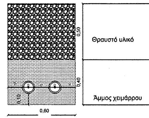
ΤΥΠΙΚΗ ΔΙΑΤΟΜΗ 3 ΟΔΕΥΣΗ ΔΥΟ ΑΓΩΓΩΝ ΕΝΤΟΣ ΟΙΚΙΣΜΟΥ ΕΠΙ ΧΑΛΙΚΟΣΤΡΩΜΕΝΗΣ ΟΔΟΥ
