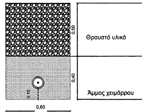
ΤΥΠΙΚΗ ΔΙΑΤΟΜΗ 3 ΟΔΕΥΣΗΣ ΑΓΩΓΟΥ ΕΝΤΟΣ ΟΙΚΙΣΜΟΥ ΕΠΙ ΧΑΛΙΚΟΣΤΡΩΜΕΝΗΣ ΟΔΟΥ
