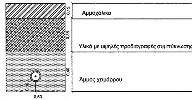
ΤΥΠΙΚΗ ΔΙΑΤΟΜΗ 6 ΟΔΕΥΣΗ ΕΝΟΣ ΑΓΩΓΟΥ ΕΚΤΟΣ ΟΙΚΙΣΜΟΥ ΕΠΙ ΧΑΛΙΚΟΣΤΡΩΜΕΝΗΣ ΑΓΡΟΤΙΚΗΣ ΟΔΟΥ
