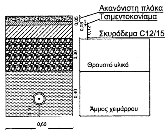
ΤΥΠΙΚΗ ΔΙΑΤΟΜΗ 5 ΟΔΕΥΣΗ ΕΝΟΣ ΑΓΩΓΟΥ ΕΝΤΟΣ ΟΙΚΙΣΜΟΥ ΕΠΙ ΠΛΑΚΟΣΤΡΩΜΕΝΗΣ ΟΔΟΥ
