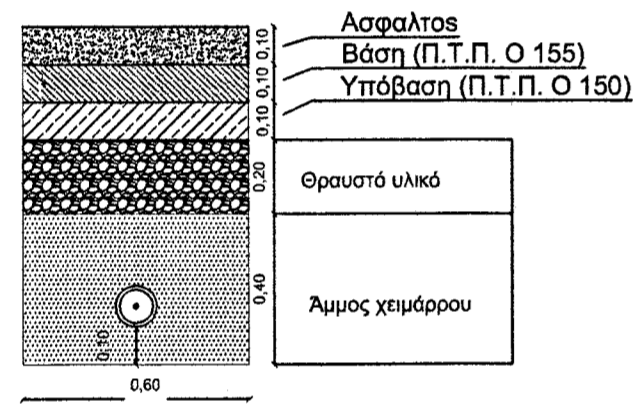
ΤΥΠΙΚΗ ΔΙΑΤΟΜΗ 1 ΟΔΕΥΣΗ ΕΝΟΣ ΑΓΩΓΟΥ ΕΝΤΟΣ ΟΙΚΙΣΜΟΥ ΕΠΙ ΑΣΦΑΛΤΟΣΤΡΩΜΕΝΗΣ ΟΔΟΥ
