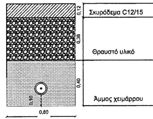
ΤΥΠΙΚΗ ΔΙΑΤΟΜΗ 2 ΟΔΕΥΣΗΣ ΑΓΩΓΟΥ ΕΝΤΟΣ ΟΙΚΙΣΜΟΥ ΕΠΙ ΤΣΙΜΕΝΟΣΤΡΩΜΕΝΗΣ ΟΔΟΥ
