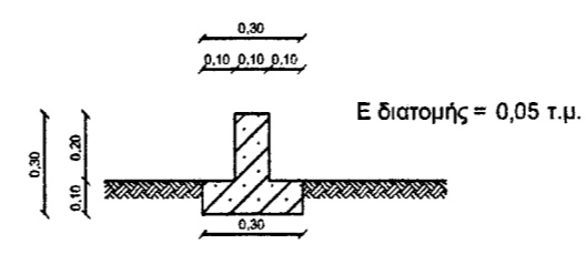
ΛΕΠΤΟΜΕΡΕΙΑ - Τομή α-α Κλίμακα 1:25
