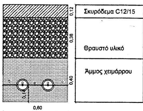
ΤΥΠΙΚΗ ΔΙΑΤΟΜΗ ΟΔΕΥΣΗΣ ΔΥΟ ΑΓΩΓΩΝ ΕΝΤΟΣ/ΕΚΤΟΣ ΟΙΚΙΣΜΟΥ ΕΠΙ ΤΣΙΜΕΝΟΣΤΡΩΜΕΝΗΣ ΟΔΟΥ
