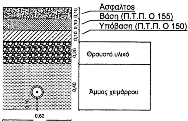
ΤΥΠΙΚΗ ΔΙΑΤΟΜΗ ΟΔΕΥΣΗ ΕΝΟΣ ΑΓΩΓΟΥ ΕΝΤΟΣ/ΕΚΤΟΣ ΟΙΚΙΣΜΟΥ ΕΠΙ ΑΣΦΑΛΤΟΣΤΡΩΜΕΝΗΣ ΟΔΟΥ
