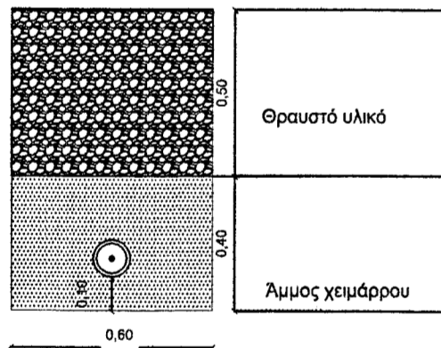
ΤΥΠΙΚΗ ΔΙΑΤΟΜΗ ΟΔΕΥΣΗΣ ΑΓΩΓΟΥ ΕΝΤΟΣ ΟΙΚΙΣΜΟΥ ΕΠΙ ΧΑΛΙΚΟΣΤΡΩΜΕΝΗΣ ΟΔΟΥ
