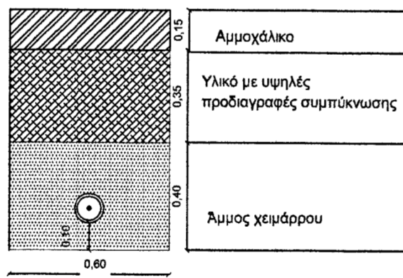
ΤΥΠΙΚΗ ΔΙΑΤΟΜΗ ΟΔΕΥΣΗ ΕΝΟΣ ΑΓΩΓΟΥ ΕΚΤΟΣ ΟΙΚΙΣΜΟΥ ΕΠΙ ΧΑΛΙΚΟΣΤΡΩΜΕΝΗΣ ΑΓΡΟΤΙΚΗΣ ΟΔΟΥ
