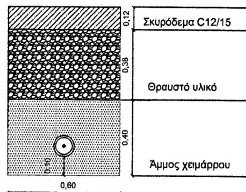
ΤΥΠΙΚΗ ΔΙΑΤΟΜΗ ΟΔΕΥΣΗΣ ΑΓΩΓΟΥ ΕΝΤΟΣ/ΕΚΤΟΣ ΟΙΚΙΣΜΟΥ ΕΠΙ ΤΣΙΜΕΝΟΣΤΡΩΜΕΝΗΣ ΟΔΟΥ
