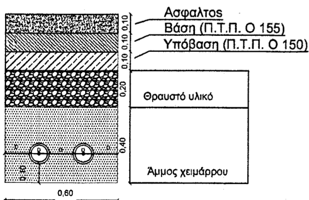
ΤΥΠΙΚΗ ΔΙΑΤΟΜΗ ΟΔΕΥΣΗ ΔΥΟ ΑΓΩΓΩΝ ΕΝΤΟΣ/ΕΚΤΟΣ ΟΙΚΙΣΜΟΥ ΕΠΙ ΑΣΦΑΛΤΟΣΤΡΩΜΕΝΗΣ ΟΔΟΥ
