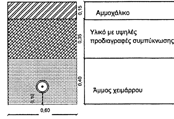
ΤΥΠΙΚΗ ΔΙΑΤΟΜΗ ΟΔΕΥΣΗ ΕΝΟΣ ΑΓΩΓΟΥ ΕΚΤΟΣ ΟΙΚΙΣΜΟΥ ΕΠΙ ΧΑΛΙΚΟΣΤΡΩΜΕΝΗΣ ΑΓΡΟΤΙΚΗΣ ΟΔΟΥ
