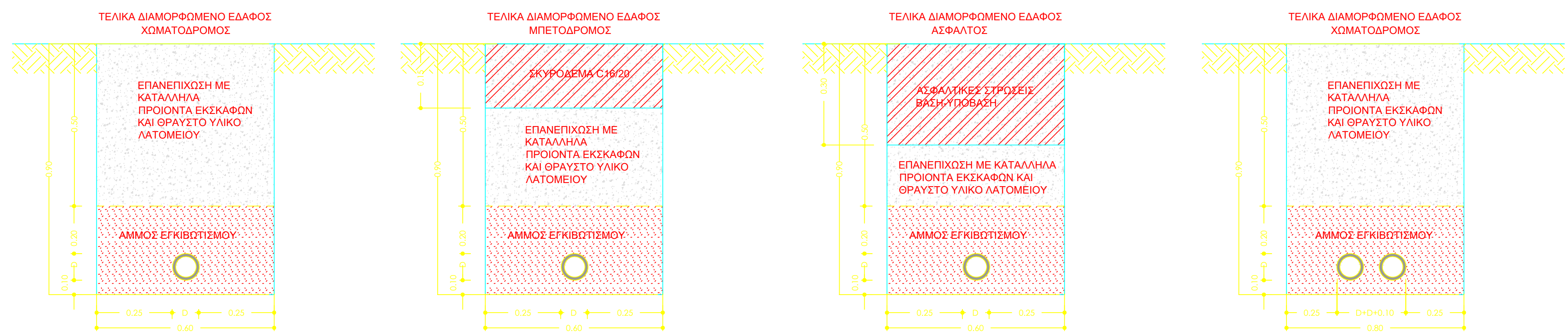
ΤΥΠΙΚΗ ΔΙΑΤΟΜΕΣ ΣΚΑΜΜΑΤΟΣ ΑΓΩΓΟΥ
